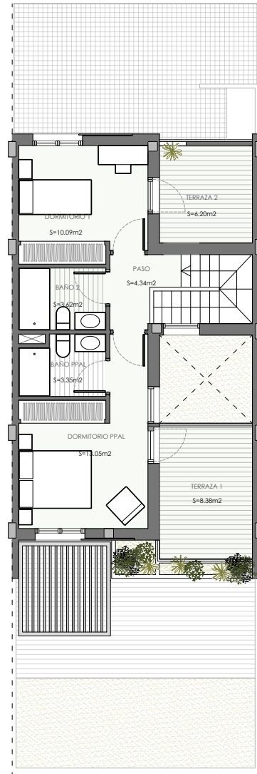
PLANTA ALTA
