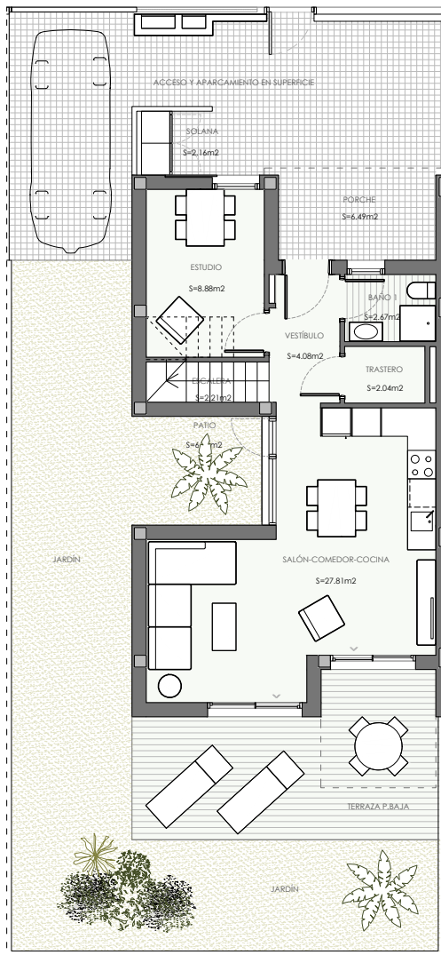
PLANTA BAJA
