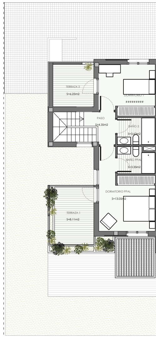
PLANTA ALTA
