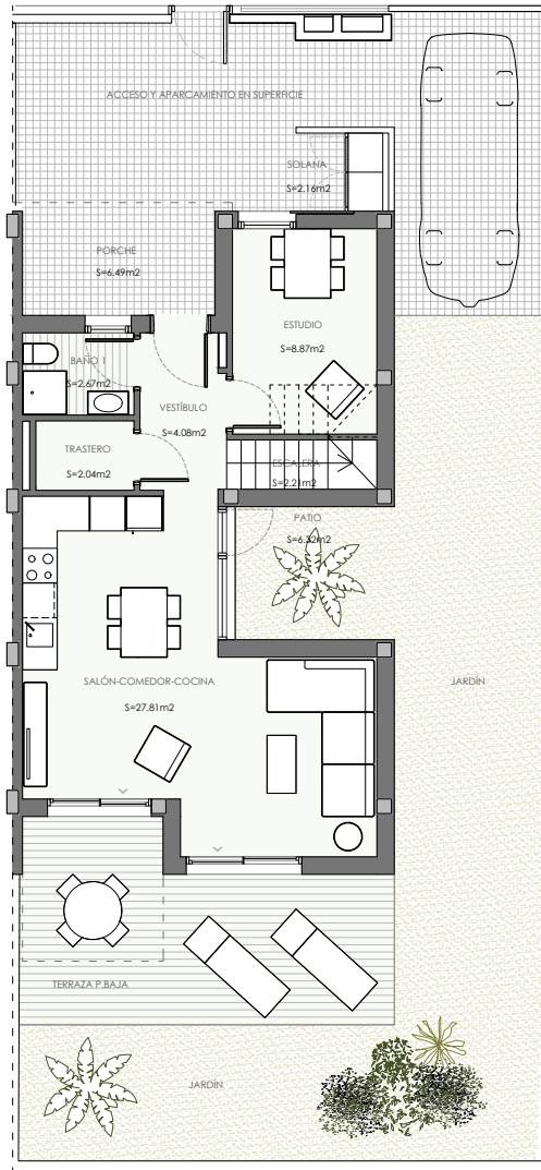
PLANTA BAJA
