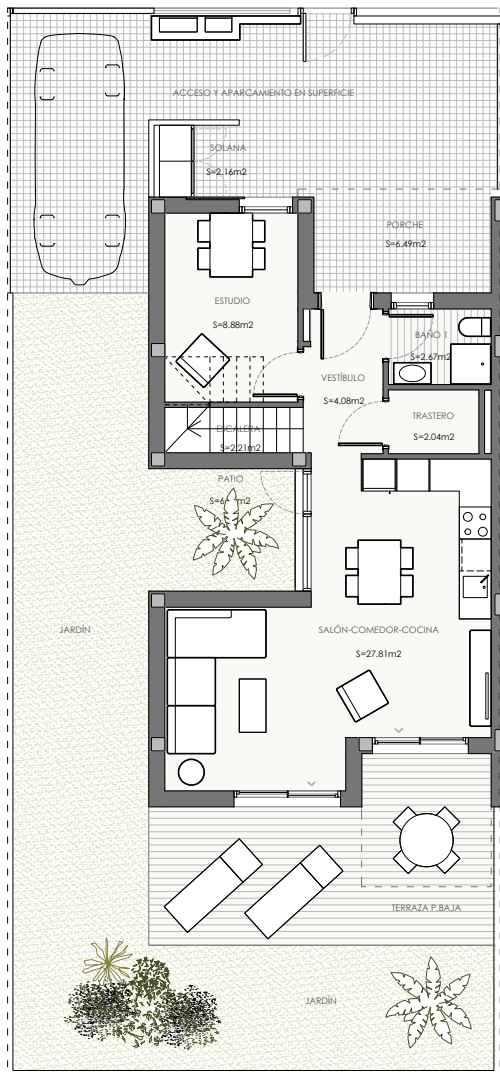
PLANTA BAJA
